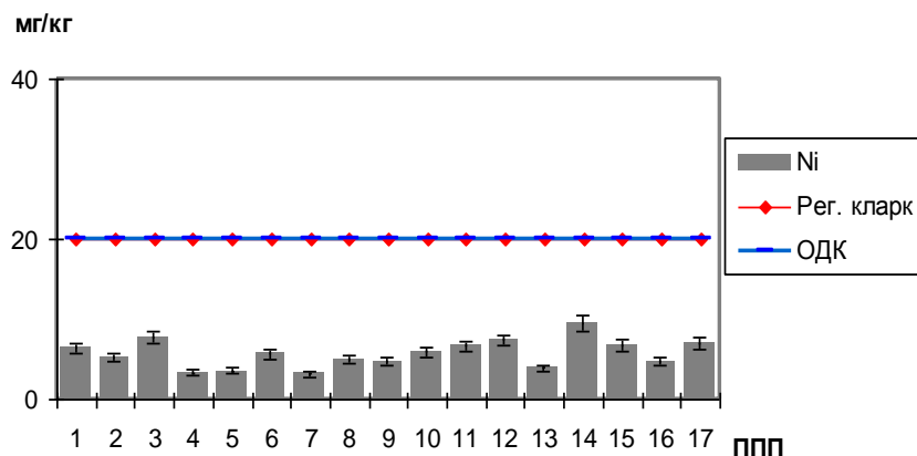
Рисунок 2 Валовое содержание Ni в дерново-подзолистой почве
