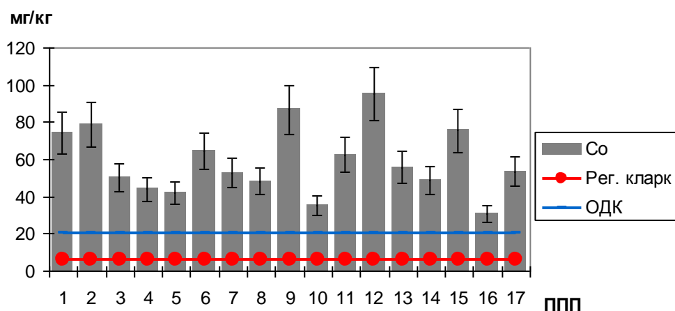
Рисунок 8 Валовое содержание Co в дерново-подзолистой почве
