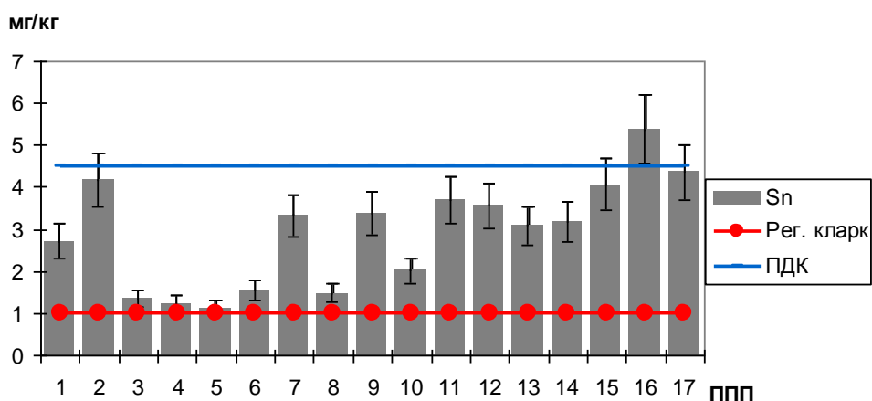
Рисунок 8 Валовое содержание Sn в дерново-подзолистой почве
