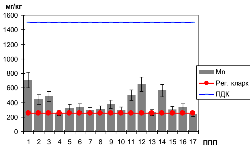
Рисунок 5 Валовое содержание Mn в дерново-подзолистой почве
