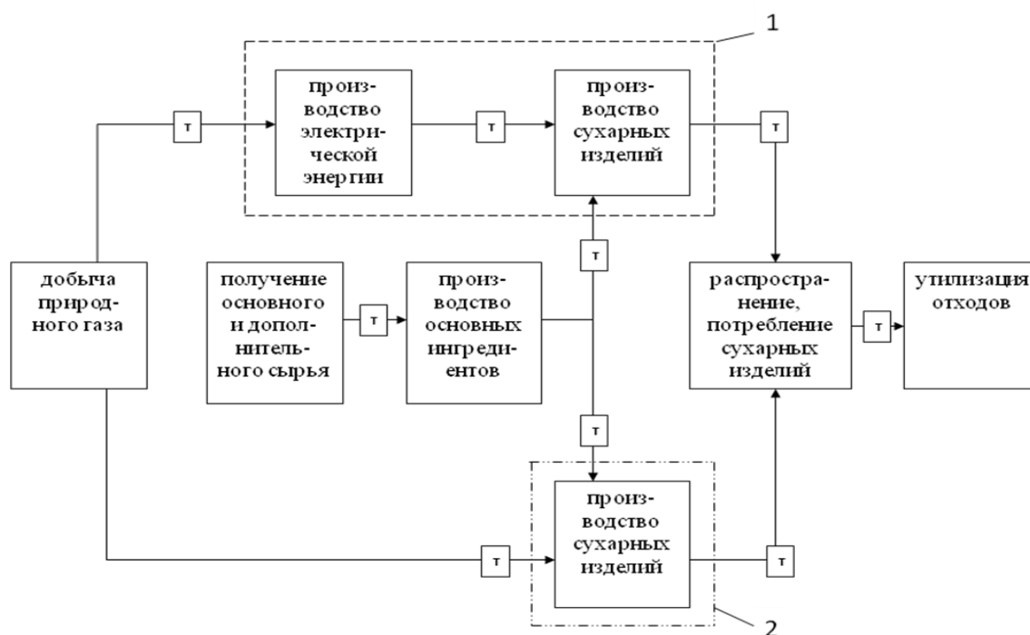
Рисунок 2 – Общая схема ЖЦ сухек: 1 – границы ПС №1; 2 – границы ПС №2
